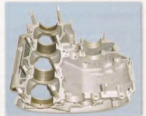
Vista de la parte superior de cárter policilíndrico
